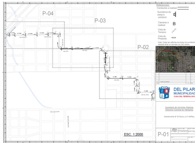
Imagen 2. Plano de planta El Roció
