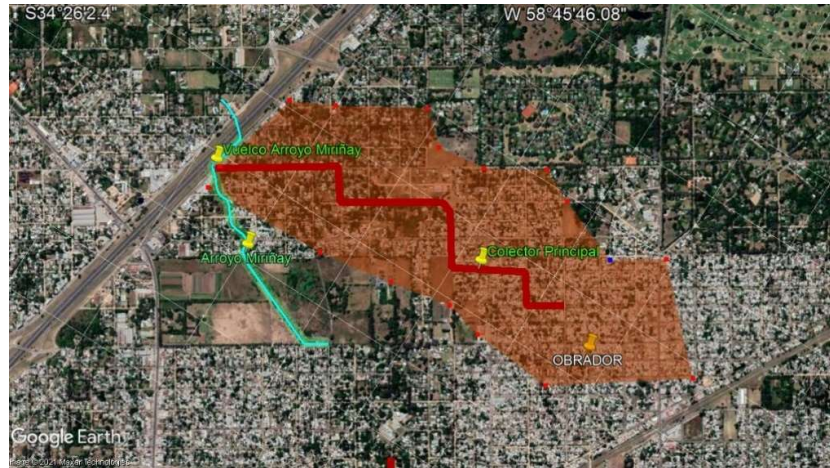
Imagen 8. Área operativa. Trazo de los conductos.
